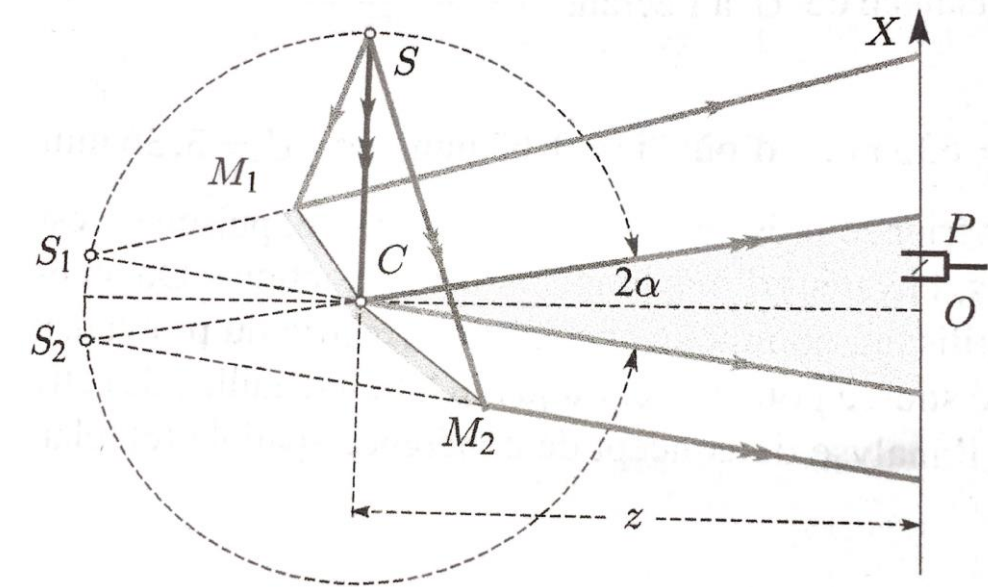
Miroirs de Fresnel
