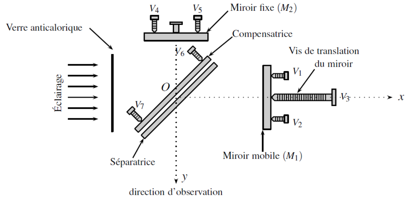
Interféromètre de Michelson
